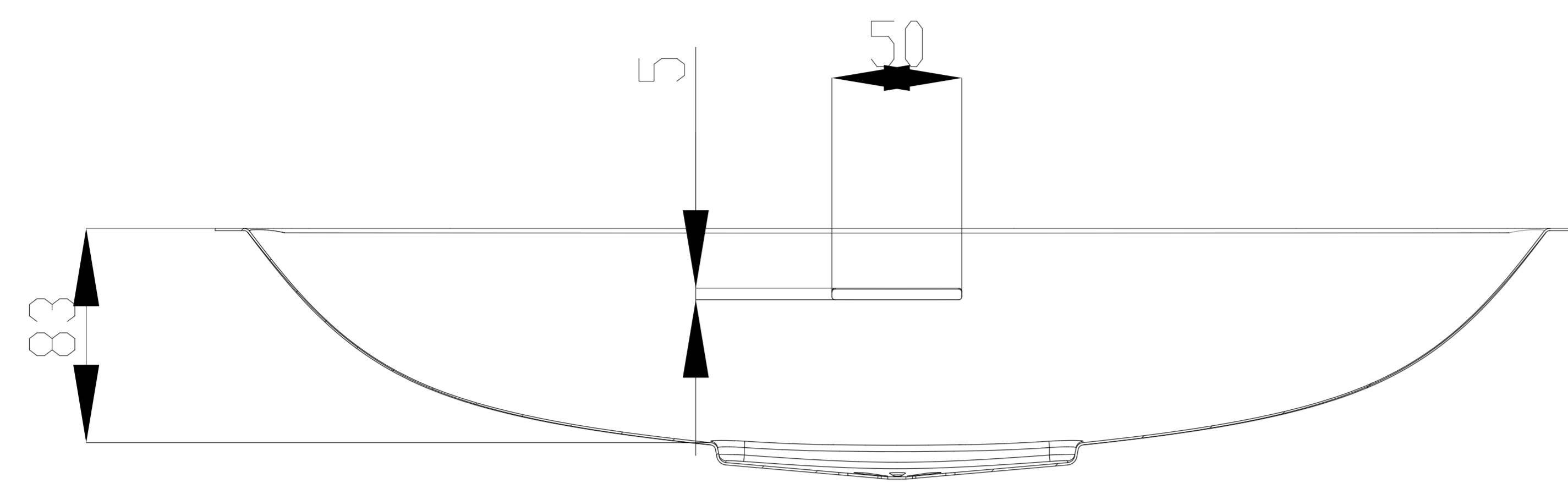
SECTION A-A
